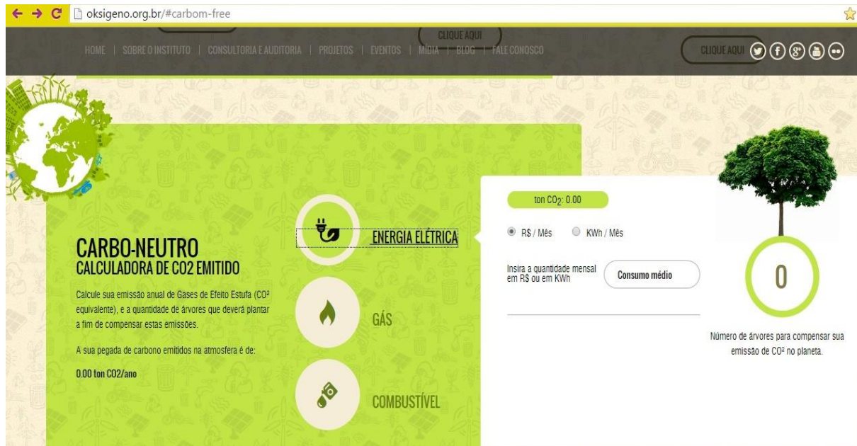
Figura 2: Cálculo de produção de CO 2 produzido pelos carros e energia elétrica.
